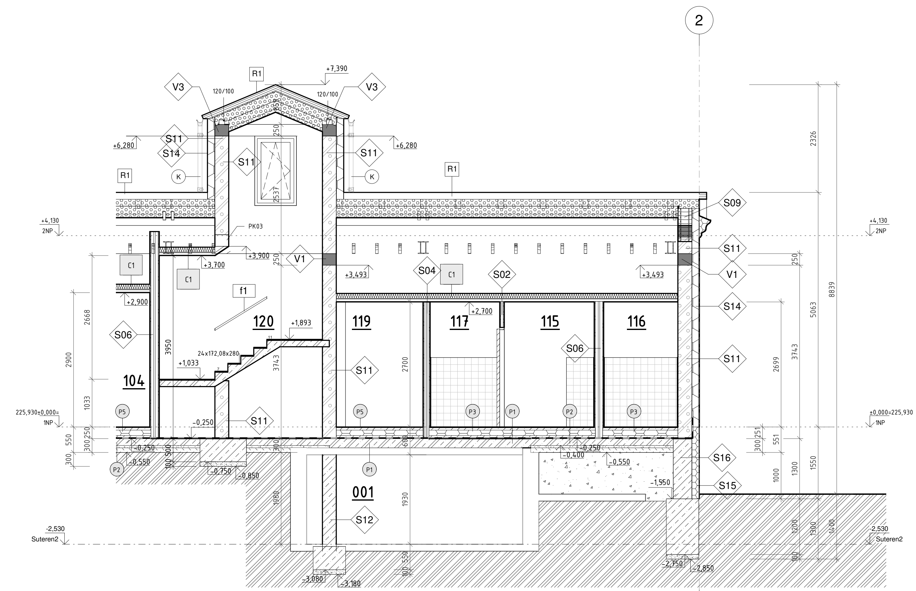
3 ŘEZ R2-R2' 1 : 50
