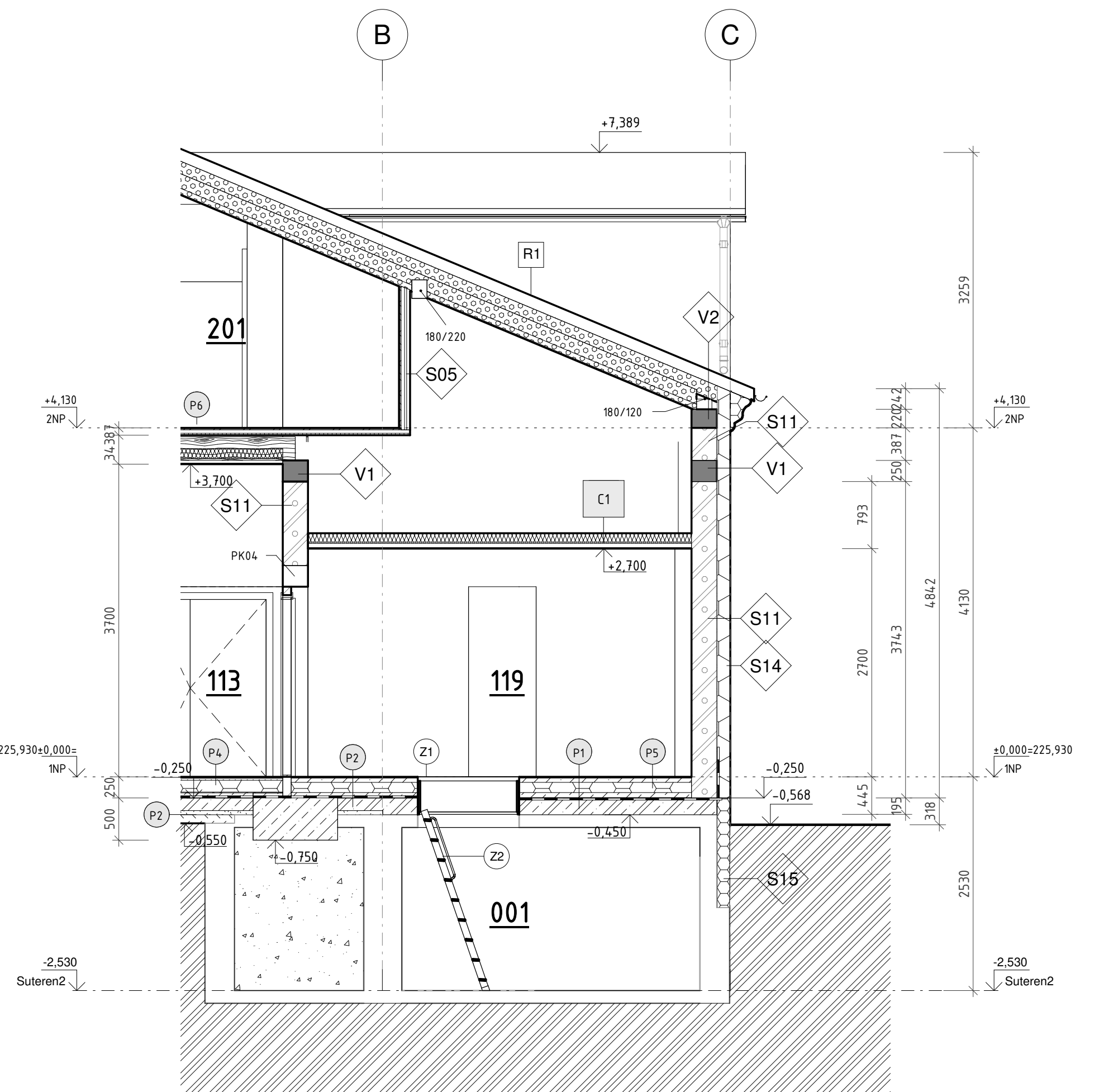
4 ŘEZ R4-R4' 1 : 50
