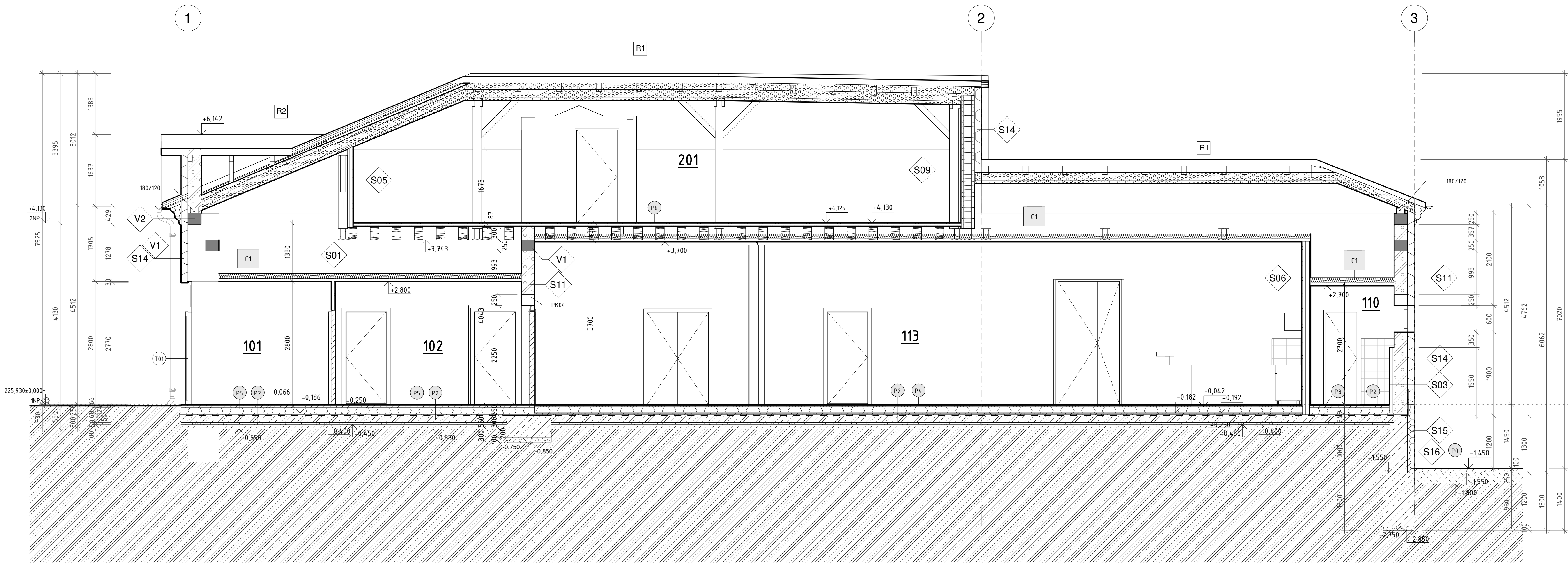
2 ŘEZ R1-R1' 1 : 50
