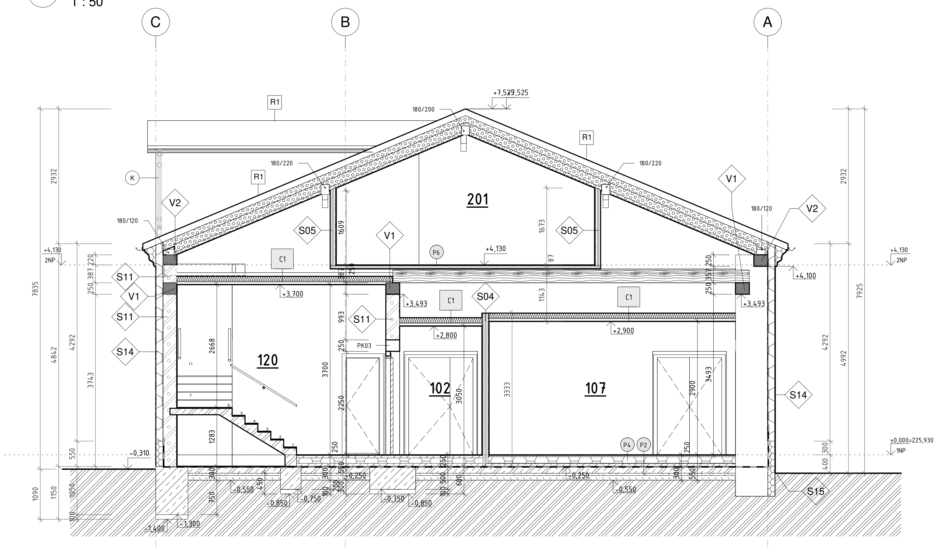
1 ŘEZ R3-R3' 1 : 50
